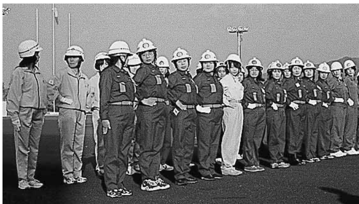
訓練式
